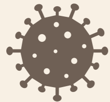
공기감염
