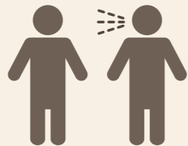
비말감염
